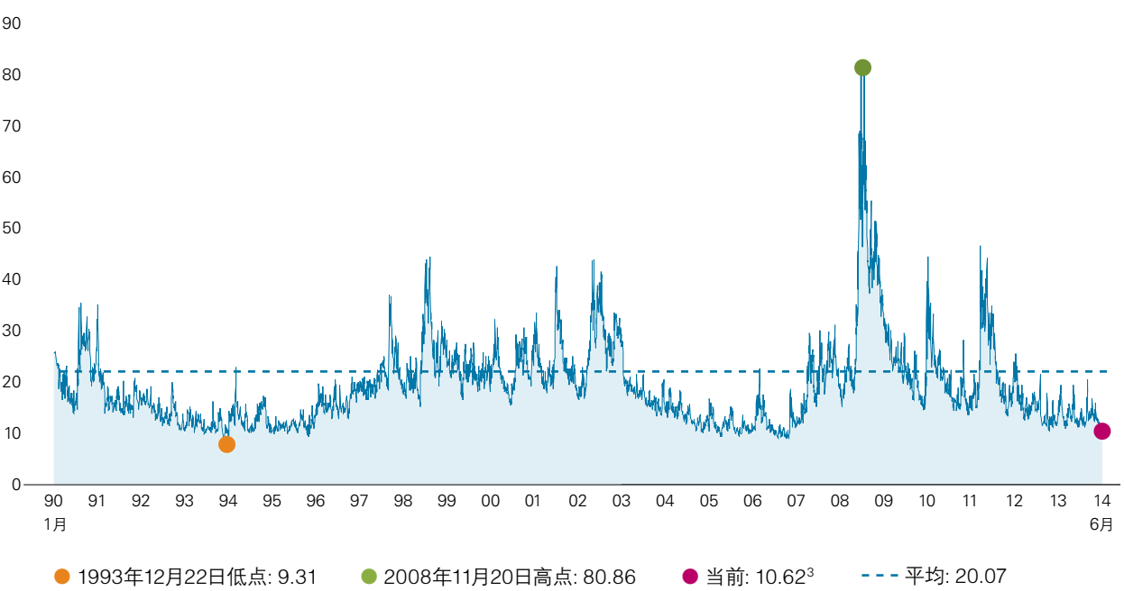
1990年1月–2014年6月的波动率指数的日趋势图
